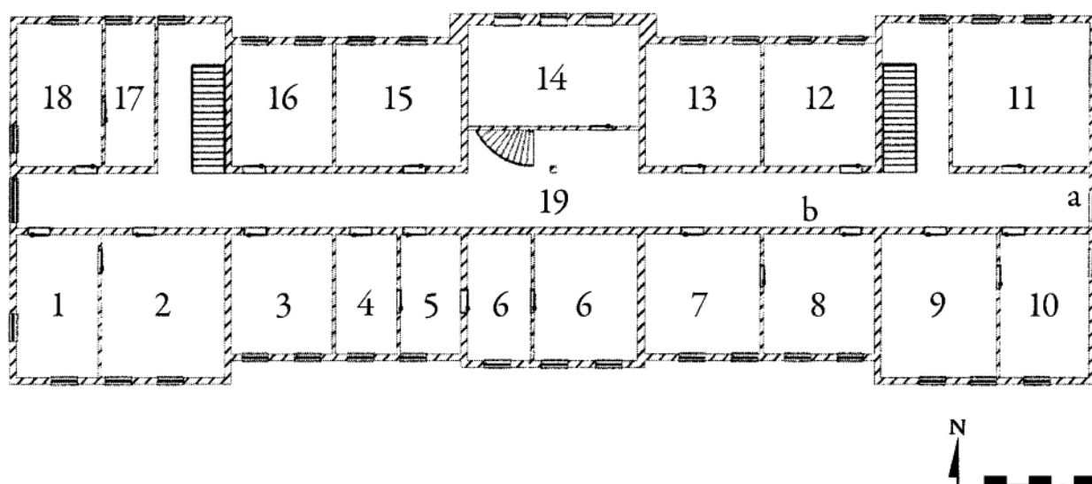
Fig. 12. Plan piętra według szkicu S. Friedberg (oprac. A. Dłuska): a – waza cloisonné; b – Carattere fiero – Anima gentile
