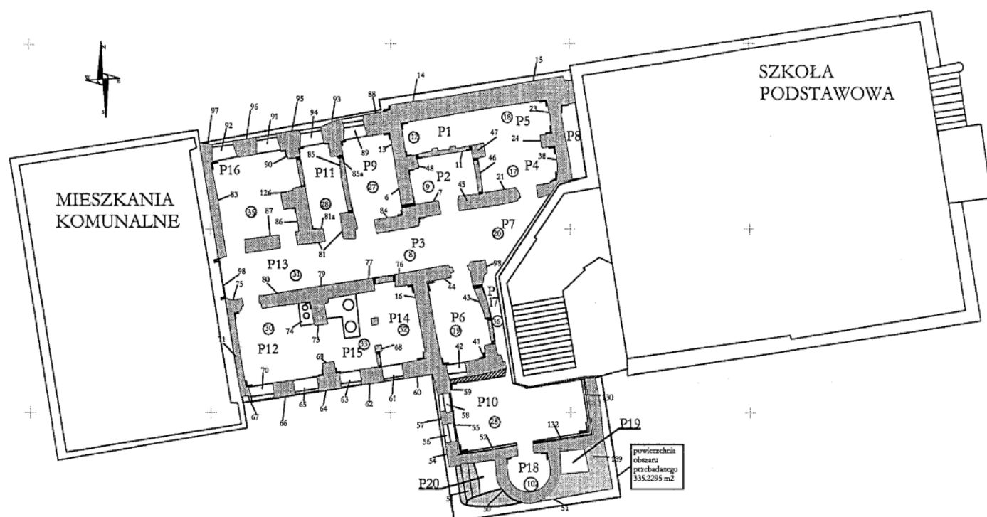
Fig. 26. Plan pomieszczeń w piwnicach dworu w Dylewie (oprac. M. Gładki)
