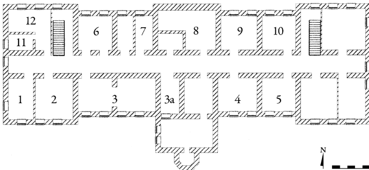
Fig. 10. Plan piwnic dworu według szkicu S. Friedberg (oprac. A. Dłuska)
