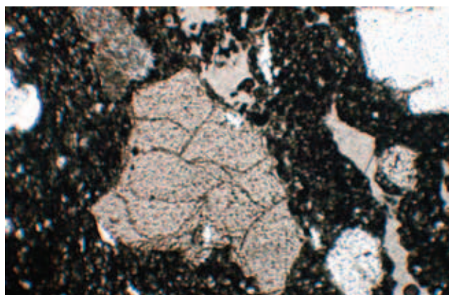
Ryc. 29. Grób 142 naczynie 3. Spękany, ostrokrawędzisty okruch kwarcu. Mikroskop polaryzacyjny, polaroid częściowo X, powiększenie 40x.
