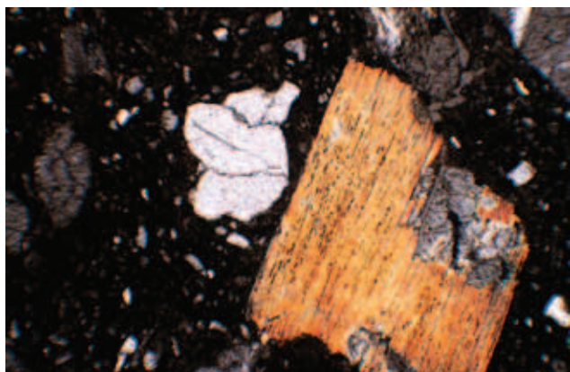
Ryc. 7. Grób 121 naczynie 3. Błazka muskowitu (mika biała) tkwiąca w masie garncarskiej. Mikroskop polaryzacyjny, polaroid częściowo X, powiększenie 40x.
