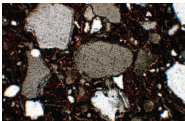
Ryc. 27. Grób 142 naczynie 1. Ostrokrawędziste (jaśnie- sze) i obtoczone (ciemniejsze) ziarna kwarcu. Mi- kroskop polaryzacyjny, polaroid częściowo X, po- większenie 40x.
