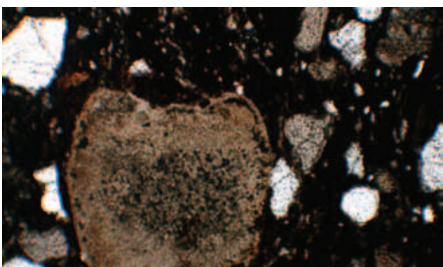
Ryc. 21. Grób 136 naczynie 2. Nierozmieszane zgrubienie materiału ilastego. Mikroskop polaryzacyjny, polaroid częściowo X, powiększenie 40x.
