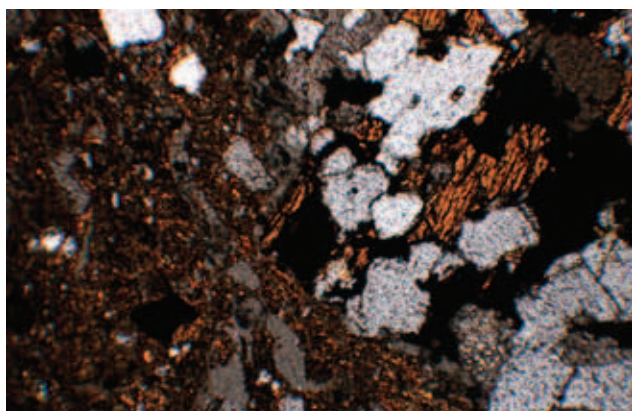
Ryc. 14. Grób 129 naczynie 1. Okruch skały magmowej, kwarcowo-skaliowej z biotytem i minerałami kruszczowymi tkwiący w masie garncarskiej. Mikroskop polaryzacyjny, polaroid częściowo X, powiększenie 40x.
