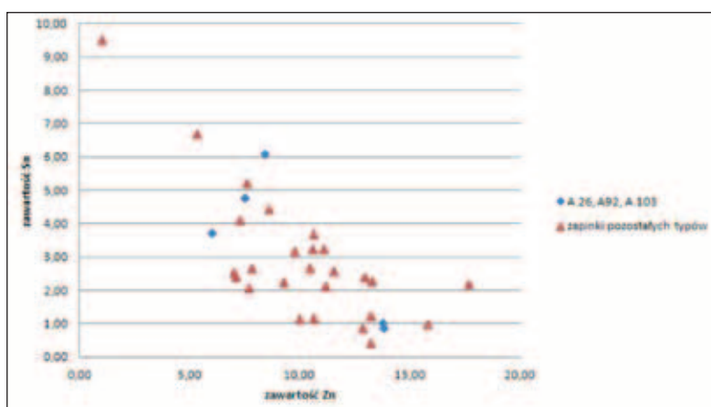
Ryc. 2. Zróżnicowanie zawartości Zn/Sn zapinek niecharakterystycznych dla kultury przeworskiej (A.26, A.92, A.103) wobec pozostałych analizowanych zapinek.
