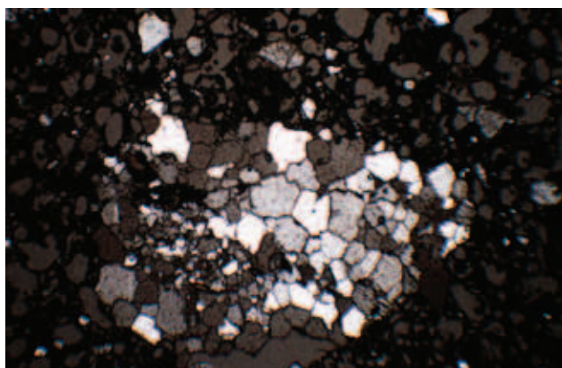
Ryc. 26. Grób 137 naczynie 3. Duży, pojedynczy okruch kwarcytu. Mikroskop polaryzacyjny, polaroid czę- ściowo X, powiększenie 40x.
