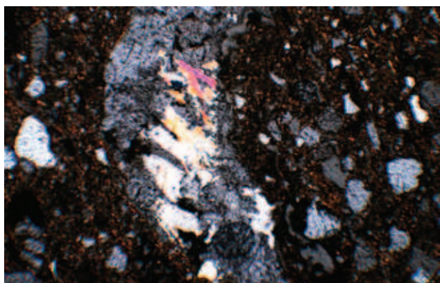
Ryc. 3. Grób 103 naczynie 1. Okrusz skały skaleniowo-tyzycykowej widoczny w masie ceramicznej. Mikroskop polaryzacyjny, polaroid częściowo X, powiększenie 40x.
