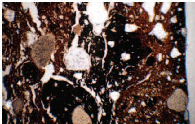
Ryc. 11. Grób 128 naczynie 1. Obraz niedokładnie zmieszanej masy ceramicznej. Widoczne zgrubienia niezmięsanego materiału powodujące pęknięcia w ściankach naczynia. Mikroskop polaryzacyjny, polaroid częściowo X, powiększenie 40x.
