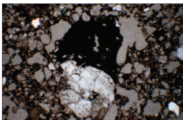
Ryc. 30. Grób 142 naczynie 5. Widoczny pojedynczy frag- ment dziegciu (czarny) z przypiętym kwaśnym plagioklazem (w paseczki). Mikroskop polaryzacyj- ny, polaroid częściowo X, powiększenie 40x.
