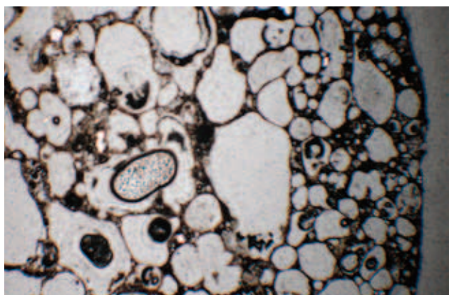
Ryc. 9. Grób 121 naczynie 5. Ziarna kwarcu związane niedużą ilością substancji wiążącej. Mikroskop polaryzacyjny, polaroid częściowo X, powiększenie 40x.
