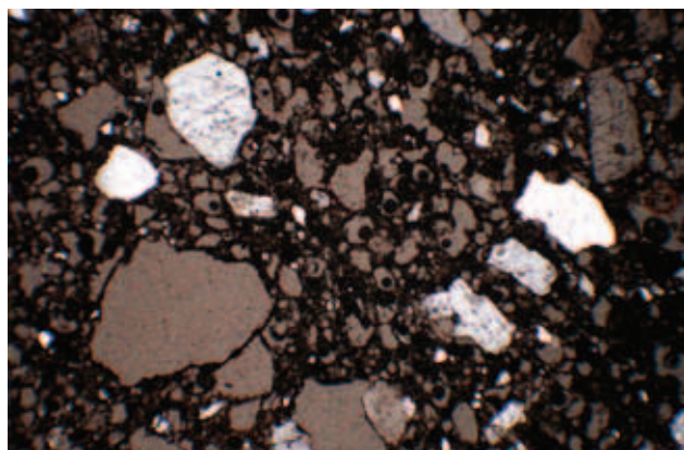
Ryc. 10. Grób 121 naczynie 8. Ziarna kwarcu i skaleni umieszczone w masie zawierającej czarny pył węglowy. Mikroskop polaryzacyjny, polaroid częściowo X, powiększenie 40x.
