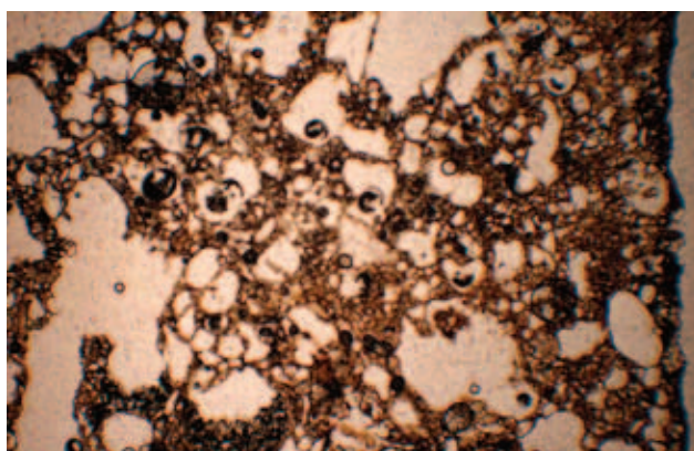
Ryc. 24 Grób 137 naczynie 1. Jasne ziarna kwarcu związane brązowym spoiwem - minerałami ilastymi z domieszką substancji smolistej – dziegciem(?) Mikroskop polaryzacyjny, jeden polaroid, powiększenie 40X.
