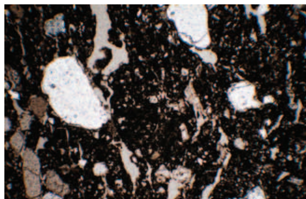
Ryc. 18. Grób 135 naczynie 3. Masa ceramiczna niedokładnie wysuszona przed wypałem, wskutek czego widoczne liczne nieregularne spękania. Mikroskop polaryzacyjny, polaroid częściowo X, powiększenie 40x.
