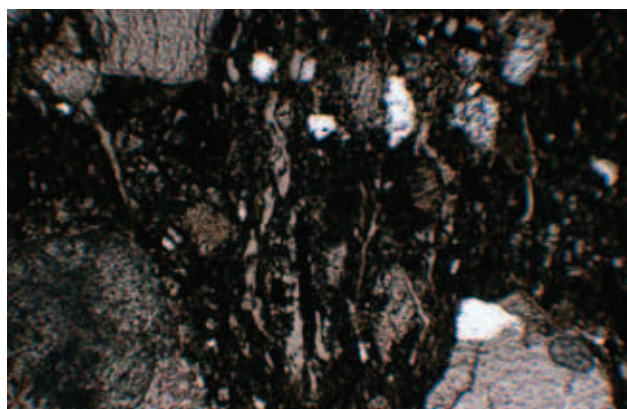
Ryc. 6. Grób 121 naczynie 2. Widoczne równoległe pęknięcia w ściankach naczynia. Mikroskop polaryzacyjny, polaroid częściowo X, powiększenie 40x.
