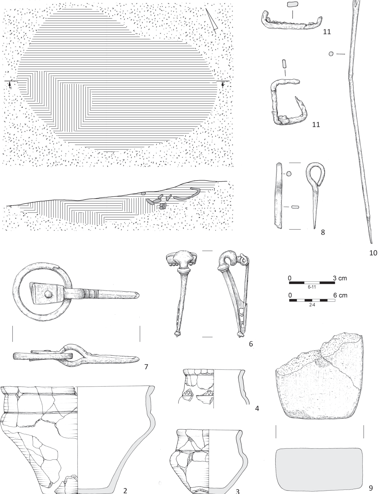
Tabl. XL. Obiekt 50: 2-4 – glina, 6 – stop miedzi, 7, 8, 10, 11 – żelazo, 9 – kamień Plate XL. Feature 50: 2-4 – clay, 6 – copper alloy, 7, 8, 10, 11 – iron, 9 – stone
