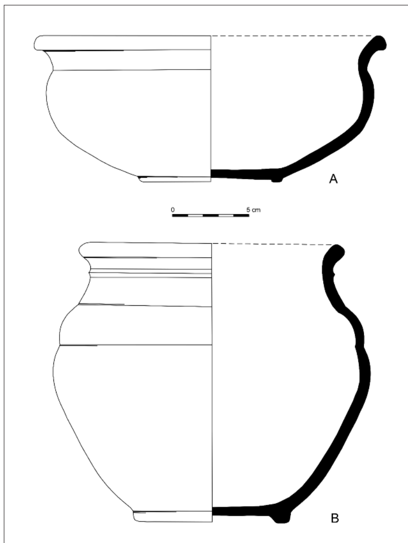
Ryc. 4. Naczynia gliniane z Baborowa (rys. P. Dulęba).
